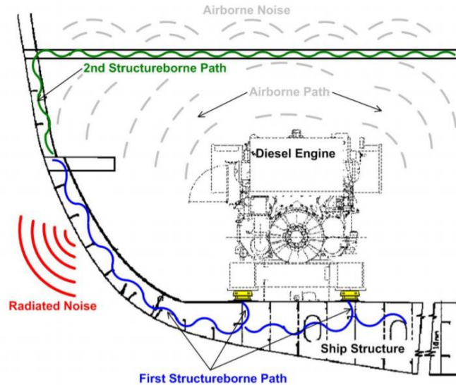
ภาพที่ 2 การส่งผ่านเสียง (ความสั่นสะเทือน) จากเครื่องยนต์ผ่านตัวเรือ 4
