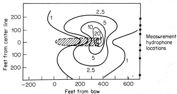
ภาพที่ 7 การแพร่ของเสียงบริเวณใ้จักรท้ายเรือ
