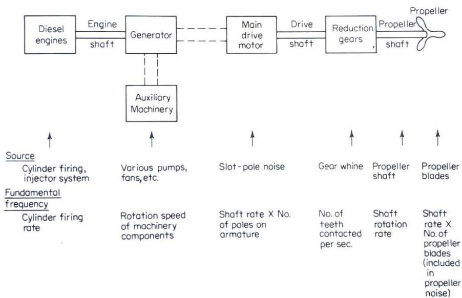
ภาพที่ 1 ส่วนประกอบของเครื่องกลและแหล่งกำเนิดเสียงที่เกิดจากเครื่องยนต์แบบ Diesel-Electric 3
