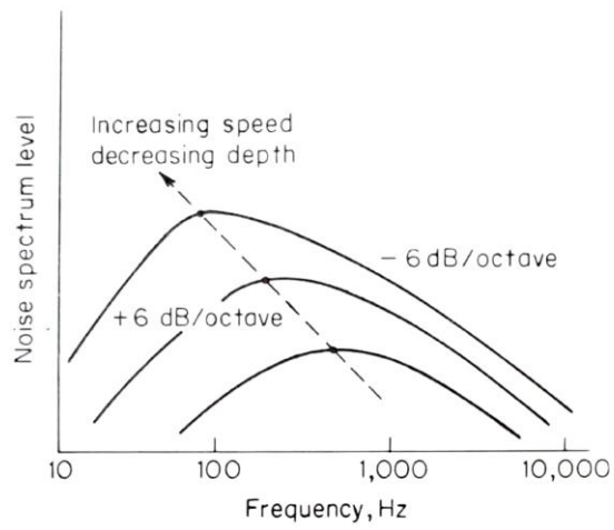
ภาพที่ 4 ความแตกต่างของการเกิดเสียงจากโพรงอากาศใบจักรที่ความเร็วและความลึกน้ำต่างกัน 6
