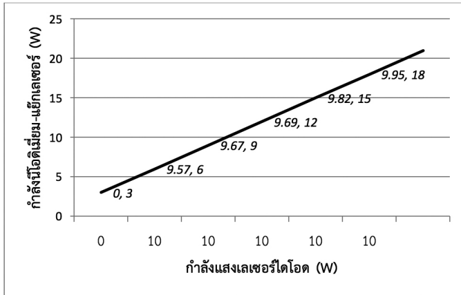
รูปที่ 10 กราฟความสัมพันธ์ระหว่างกำลังเลเซอร์ไดโอดขนาด 40 W กับกำลังมีโอติเมียมแยมิกเลเซอร์
