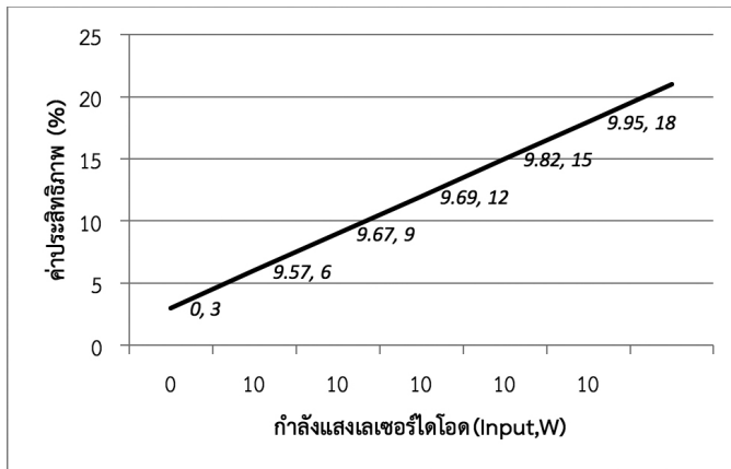
รูปที่ 11 กราฟแสดงประสิทธิภาพของระบบนีโอติเมียมแยมิกเลเซอร์ (Output, W) กับกำลังแสงที่กระตุ้นจากเลเซอร์ไดโอด 20 W (Input, W)
