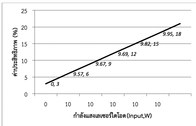
รูปที่ 12 กราฟแสดงประสิทธิภาพของระบบนีโอติเมียมแยมิกเลเซอร์ (Output,W) กับกำลังแสงที่กระตุ้นจากเลเซอร์ไดโอด 40 W (Input,W)
