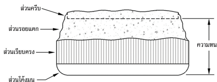
รูปที่ 4 ลักษณะส่วนประกอบของขอบตัดแผ่นเปล่า (Blank) ชิ้นงานโลหะแผ่น [11]
