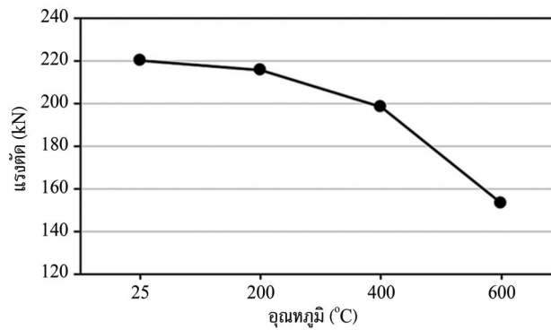
รูปที่ 8 ความสัมพันธ์ของอุณหภูมิและแรงในการบีบอัดโลหะแผ่น
