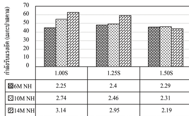
รูปที่ 3 กำลังรับแรงดัดของคานคอนกรีตเมื่อใช้จีโอโพลิเมอร์มอร์ตาร์เป็นวัสดุซ่อมอุดที่อายุ 28 วัน
