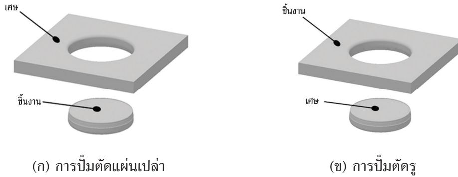
รูปที่ 1 การปั๊มตัดโลหะแผ่น
