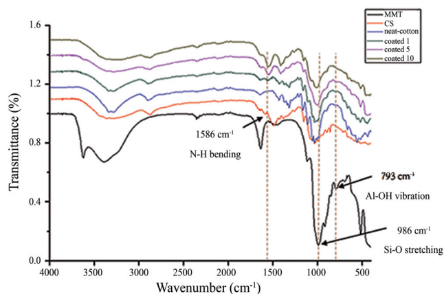
รูปที่ 1 FT-IR Spectra ของมอนต์มอริลโลไนต์ (MMT) โคโคซาน (CS) ผ้าฝ้ายที่ไม่ผ่านการเคลือบ (Neat-Cotton) และผ้าฝ้ายที่ผ่านการเคลือบด้วยคอมพอลิบบน 1 รอบ (Coated 1) 5 รอบ (Coated 5) และ 10 รอบ (Coated 10)
