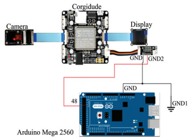
(ก) วงจรสำหรับตรวจจับหน้ากาคนามัย
