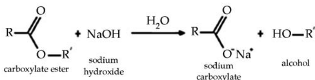
รูปที่ 2 ปฏิกิริยาไฮโดรไลซิสด้วยโซเดียมไฮดรอกไซด์
