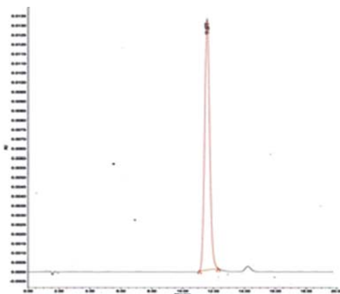
รูปที่ 3 โครมาโทแกรมของสารละลายมาตรฐานกรดเพรูลิกเข้มข้น 50 มิลลิกรัมต่อลิตร โดยเฟสเคลื่อนที่ สารละลายผสมเมทานอลต่อกรดอะซิติกเข้มข้นร้อยละ 1 อัตราส่วน 30 ต่อ 70
