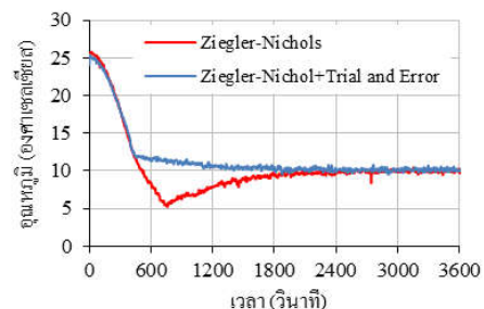
รูปที่ 12 ผลตอบสนองของระบบควบคุมเมื่อทำการตั้งค่าเป้าหมายที่ 10 องศาเซลเซียส
