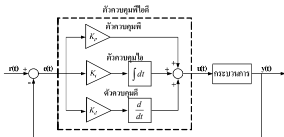
รูปที่ 1 รูปแบบโดยทั่วไปของระบบควบคุมแบบพีไอดี
