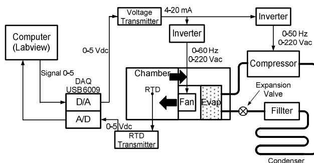
รูปที่ 5 ระบบควบคุมของเครื่องทำความเย็น
