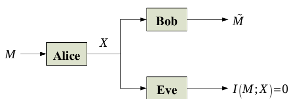
รูปที่ 1: ระบบความลับของ Shannon
