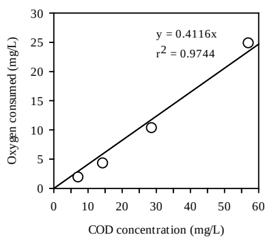
รูปที่ 6 ความสัมพันธ์เชิงเส้นตรงเฉลี่ยความเข้มข้นตัวอย่างสลัดจ์ 4,081 \pm 71 มิลลิกรัม/ลิตร
