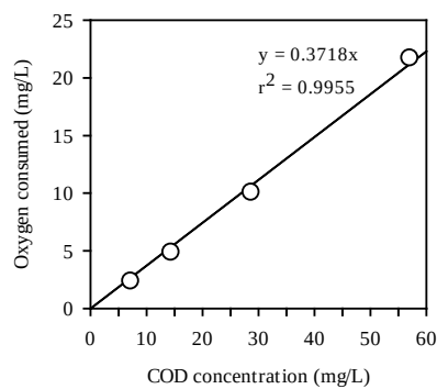
รูปที่ 4 ความสัมพันธ์เชิงเส้นตรงเฉลี่ยความเข้มข้นตัวอย่างสลัดจ์ 2,186 \pm 27 มิลลิกรัม/ลิตร
