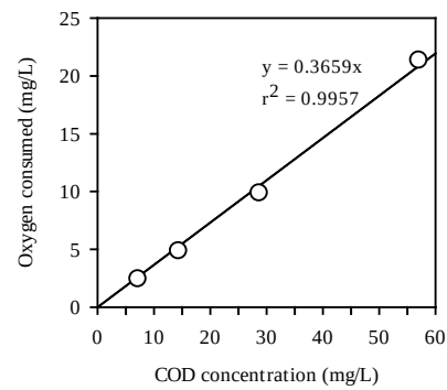
รูปที่ 3 ความสัมพันธ์เชิงเส้นตรงเฉลี่ยความเข้มข้นตัวอย่างสลัดจ์ 880 \pm 112 มิลลิกรัม/ลิตร
