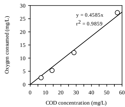
รูปที่ 5 ความสัมพันธ์เชิงเส้นตรงเฉลี่ยความเข้มข้นตัวอย่างสลัดจ์ 3,002 \pm 84 มิลลิกรัม/ลิตร
