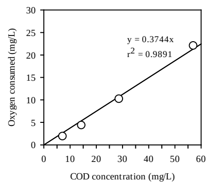
รูปที่ 7 ความสัมพันธ์เชิงเส้นตรงเฉลี่ยความเข้มข้นตัวอย่างสลัดจ์ 5,297 \pm 61 มิลลิกรัม/ลิตร
