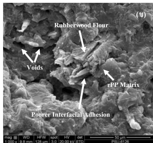
รูปที่ 2 โครงสร้างพื้นฐานวิทยาของวัสดุเชิงประกอบพอลิโพรพิลีนรีไซเคิลที่เติมผงไม้ยางพารา (ก) 25% และ (ข) 45% ที่กำลังขยาย 1000×
