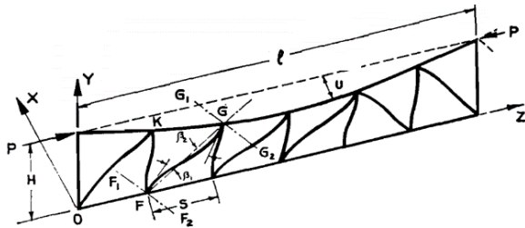
รูปที่ 1 รูปแบบการเลี้ยวรูปของโครงถัก [4]
