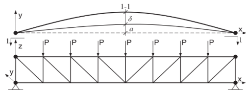
รูปที่ 4 การเลี้ยวรูปของชิ้นส่วนภายใต้แรงกระทำ [6]
