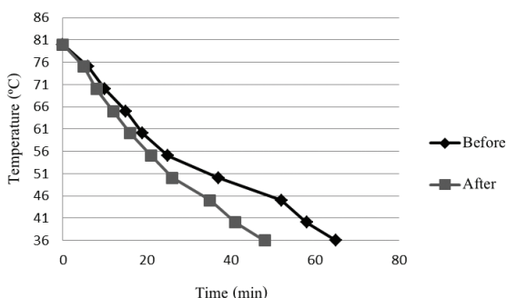
รูปที่ 8 ความสัมพันธ์ระหว่างอุณหภูมิถึงผสมและเวลาที่ใช้ของสภาวะก่อนและหลังการปรับปรุงกระบวนการ
