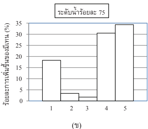
รูปที่ 5 ร้อยละของการเพิ่มขึ้นของมีเทนที่ปริมาตรน้ำร้อยละ 25 และ 75 ของปริมาตรถึง Scrubber ที่เงื่อนไขการทดลองต่างๆ
