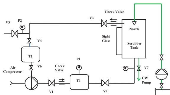
รูปที่ 4 แผนผังอุปกรณ์การทดลอง
