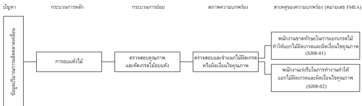
รูปที่ 6 แผนผังต้นไม้แสดงสาเหตุของปัญหาข้อมูลปริมาณการผลิตคลาดเคลื่อนสำหรับกระบวนการอบแห้งไม้
