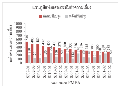
รูปที่ 9 ผลการประเมิน FMEA เปรียบเทียบก่อนและหลังการปรับปรุง
