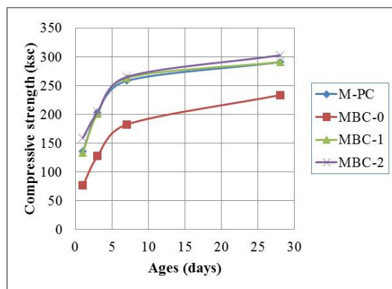
รูปที่ 2 ความสัมพันธ์ระหว่างกำลังอัดและอายุการบ่มของมอร์ตาร์ผสมหินฝุ่นแทนทราย
