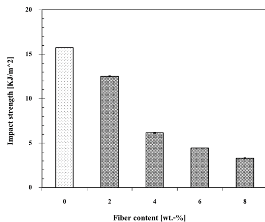
รูปที่ 6 แสดงค่าความต้านทานการกระแทกของวัสดุคอมโพสิตเทอร์โมพลาสติกสตาซจากแป้งดัดแปรที่เติมเส้นใยไบสับปะรดอัตราส่วนต่างๆ
