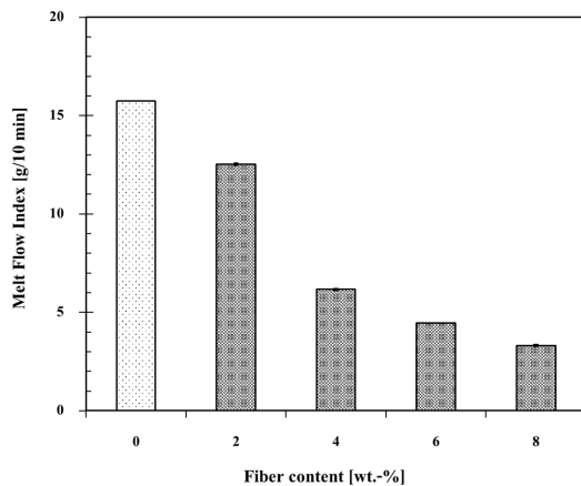
รูปที่ 7 แสดงค่าดัชนีการไหลของวัสดุคอมโพลีสเตอร์โมพลาสติกสตาซจากแป้งดัดแปรที่เติมเส้นใยไบสับประรดอัตราส่วนต่างๆ
