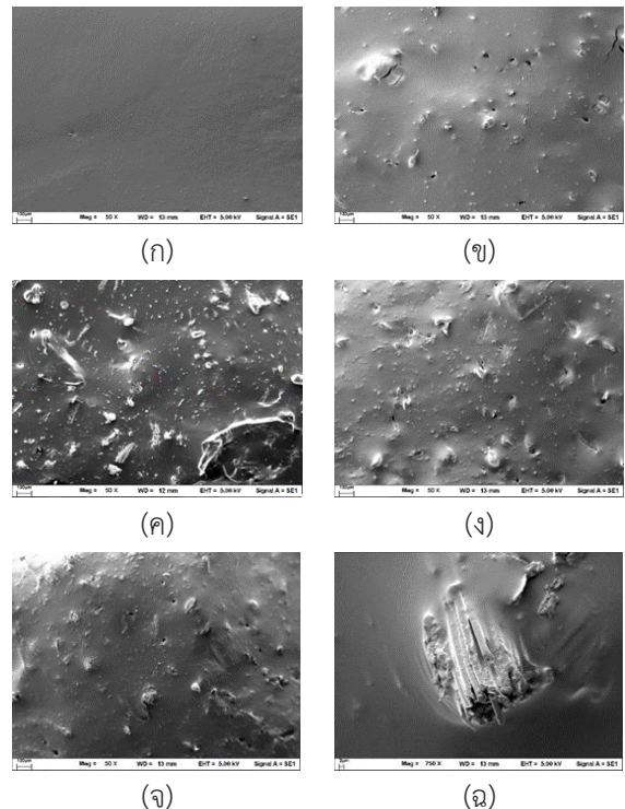
รูปที่ 8 SEM Micrograph ของคอมโพลีสเตอร์โมพลาสติกสตาซจากแป้งดัดแปรที่อัตราส่วนการผสมเส้นใยไบสับประรดที่ (ก) 0 (ข) 2 (ค) 4 (ง) 6 และ (จ) 8 phr ที่กำลังขยาย 50x ตามลำดับ และ (ฉ) คอมโพลีสเตอร์โมพลาสติกสตาซจากแป้งดัดแปรที่เติมเส้นใยไบสับประรดที่ 8 phr ที่กำลังขยาย 750x
