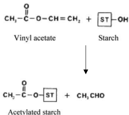
รูปที่ 1 ปฏิกิริยาเอซิติลเลชันระหว่างแป้งกับไวน์ลแอซิเตท [17]
