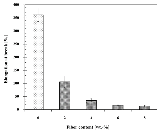
รูปที่ 5 แสดงค่าร้อยละการยืด ณ จุดขาดของวัสดุคอมโพสิตเทอร์โมพลาสติกสตาซจากแป้งดัดแปรที่เติมเส้นใยไบสับปะรดอัตราส่วนต่างๆ
