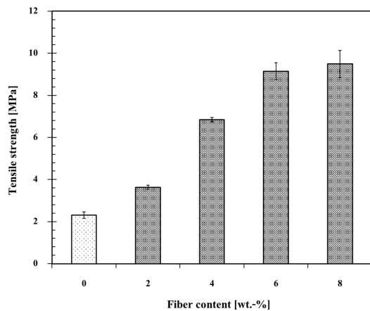
รูปที่ 3 แสดงค่าความต้านทานแรงดึงของวัสดุคอมโพสิตเทอร์โมพลาสติกสตาซจากแป้งดัดแปรที่เติมเส้นใยไบสับปะรดอัตราส่วนต่างๆ
