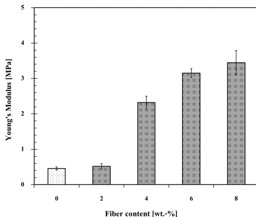
รูปที่ 4 แสดงค่ายังส์มอดุลัสของวัสดุคอมโพสิตเทอร์โมพลาสติกสตาซจากแป้งดัดแปรที่เติมเส้นใยไบสับปะรดอัตราส่วนต่างๆ
