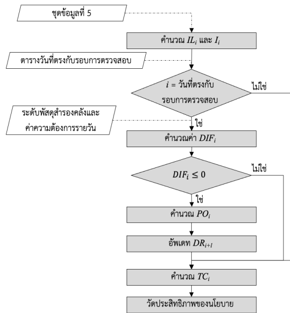
รูปที่ 4 ขั้นตอนการกำหนดและทดสอบนโยบายการเติมเต็มพัสดุคลังแบบพอดีกับความต้องการในแต่ละคาบ
