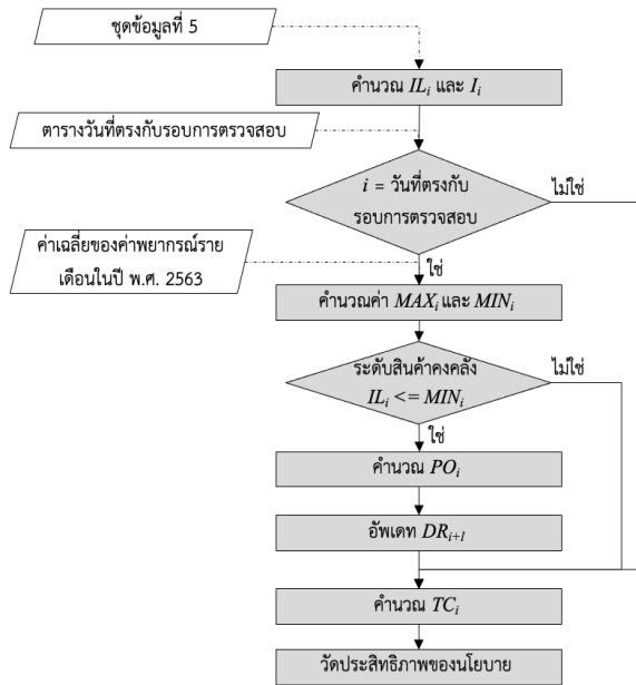
รูปที่ 3 ขั้นตอนการกำหนดและทดสอบนโยบายการเติมเต็มพัสดุคงคลังแบบเติมเต็มค่าสูงสุดต่ำสุด (Max-Min)
