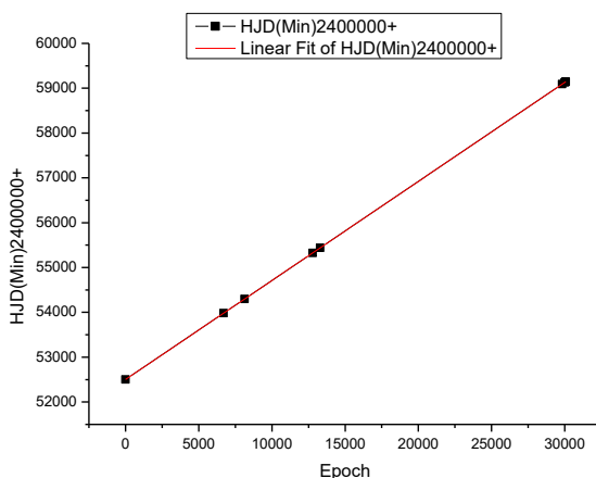
รูปที่ 1 กราฟความสัมพันธ์ระหว่างค่ายุคกับค่าเวลาที่แสงน้อยที่สุด (HJD)
