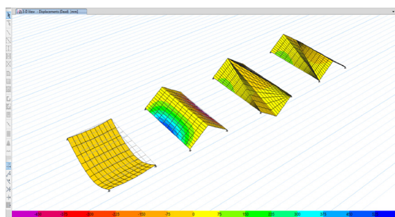
รูปที่ 8 ลักษณะการแอ่นตัว ของแผ่นพับแบบเดี่ยว
