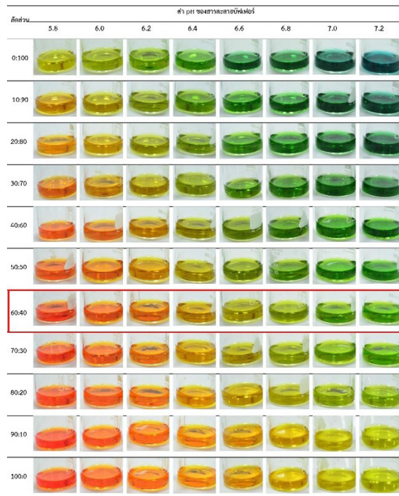
รูปที่ 2 การเปลี่ยนแปลงสีของสารละลายอินดิเคเตอร์ผสมระหว่าง Methyl Red และ Bromothymol Blue ที่อัตราส่วนต่างๆ ปริมาตร 0.30 มิลลิลิตร ในสารละลายบัฟเฟอร์ที่ค่าความเป็นกรด-ด่างในช่วง 5.8-7.2
