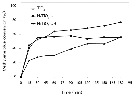
รูปที่ 5 ร้อยละการเปลี่ยนของเมทิลีนบลูในปฏิกิริยาโฟโตคะตะไลติกภายใต้แสงวิสิเบิลของตัวเร่งปฏิกิริยา \text{TiO}_2 , \text{N/TiO}_2\text{-UL} และ \text{N/TiO}_2\text{-UH}
