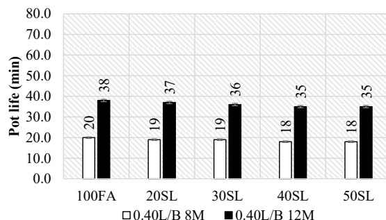
รูปที่ 13 ค่าระยะเวลาในการทำงานของวัสดุเชื่อมประสานกระตุ้นด้วยต่างจากเถ้าลอยแทนที่ด้วยเถ้าตะกอนเหล็กที่อัตราส่วนของเหลวต่อวัสดุประสานเท่ากับ 0.40 และแปรผันความเข้มข้นของสารละลาย NaOH
