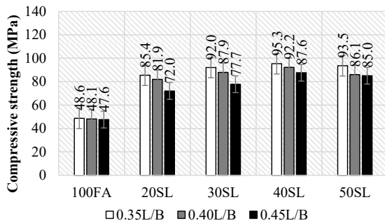
รูปที่ 8 กำลังรับแรงอัดของวัสดุเชื่อมประสานกระตุ้นด้วยต่างจากเถาลอยแทนที่ด้วยเถาตะกรันเหล็กที่ความเข้มข้น NaOH เท่ากับ 12 โมลาร์ และแปรผันอัตราส่วนของเหลวต่อวัสดุประสานที่อายุบ่ม 28 วัน
