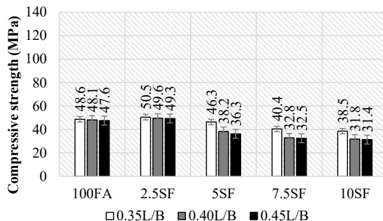
รูปที่ 7 กำลังรับแรงอัดของวัสดุเชื่อมประสานกระตุ้นด้วยต่างจากเถ้าลอยแทนที่ด้วยซิลิกาฟุ้งที่ความเข้มข้น NaOH เท่ากับ 12 โมลาร์ และแปรผันอัตราส่วนของเหลวต่อวัสดุประสานที่อายุบ่ม 28 วัน
