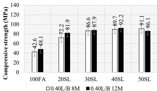
รูปที่ 14 กำลังรับอัดของวัสดุเชื่อมประสานกระตุ้นด้วยต่างจากเถ้าลอยแทนที่ด้วยเถ้าตะกอนเหล็กที่อัตราส่วนของเหลวต่อวัสดุประสานเท่ากับ 0.40 และแปรผันความเข้มข้นของสารละลาย NaOH
