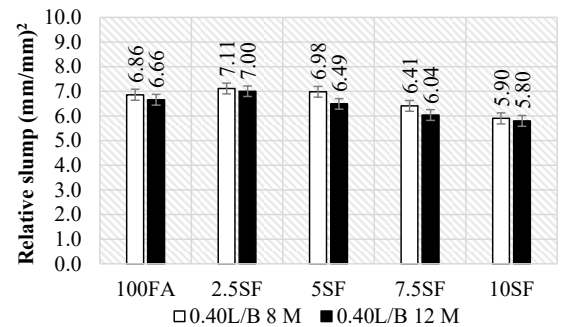
รูปที่ 9 การยุบตัวสัมพัทธ์ของวัสดุเชื่อมประสานกระตุ้นด้วยต่างเถาลอยแทนที่ด้วยซิลิกาฟุ่มที่อัตราส่วนของเหลวต่อวัสดุประสานเท่ากับ 0.40 และแปรผันความเข้มข้นของสารละลาย NaOH
