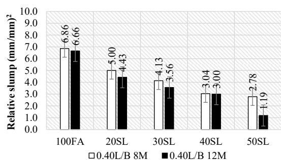
รูปที่ 12 การยุบตัวสัมพัทธ์ของวัสดุเชื่อมประสานกระตุ้นด้วยต่างจากเถ้าลอยแทนที่ด้วยเถ้าตะกอนเหล็กที่อัตราส่วนของเหลวต่อวัสดุประสานเท่ากับ 0.40 และแปรผันความเข้มข้นของสารละลาย NaOH
