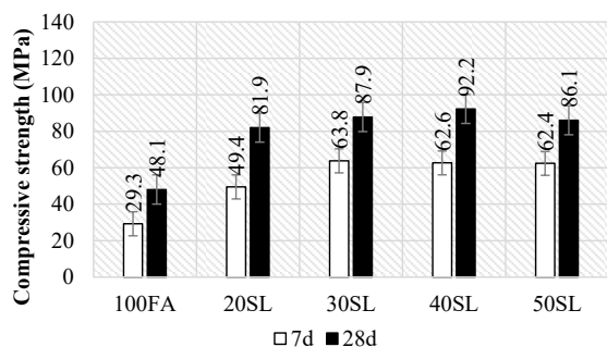
รูปที่ 6 กำลังรับแรงอัดของวัสดุเชื่อมประสานกระตุ้นด้วยต่างมอร์ตาร์จากเถ้าลอยแทนที่ด้วยเถ้าตะกอนเหล็กที่อัตราส่วนของเหลวต่อวัสดุประสานเท่ากับ 0.40 และความเข้มข้นของ NaOH เท่ากับ 12 โมลาร์
