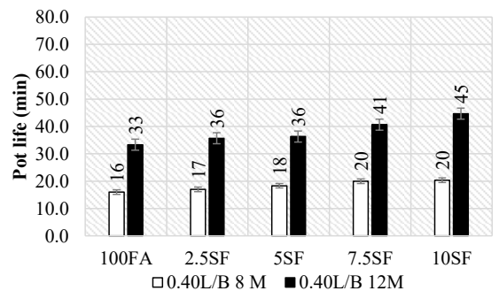
รูปที่ 10 ค่าระยะเวลาในการทำงานของวัสดุเชื่อมประสานกระตุ้นด้วยต่างจากเถาลอยแทนที่ด้วยซิลิกาฟุ่มที่อัตราส่วนของเหลวต่อวัสดุประสานเท่ากับ 0.40 และแปรผันความเข้มข้นของสารละลาย NaOH
