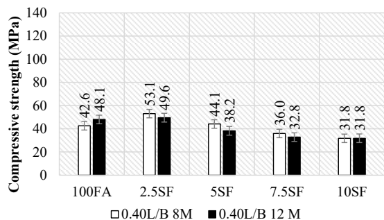
รูปที่ 11 กำลังรับแรงอัดของวัสดุเชื่อมประสานกระตุ้นด้วยต่างจากเถ้าลอยแทนที่ด้วยเถ้าตะกอนเหล็กที่อัตราส่วนของเหลวต่อวัสดุประสานเท่ากับ 0.40 และแปรผันความเข้มข้นของสารละลาย NaOH
