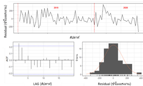
รูปที่ 12 การทดสอบ Residual ของแบบพยากรณ์ Practical
