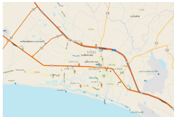
รูปที่ 1 จุดสำรวจปริมาณจราจรทั้ง 7 จุด บนถนนสายหลัก สายรองและสายท้องถิ่น
