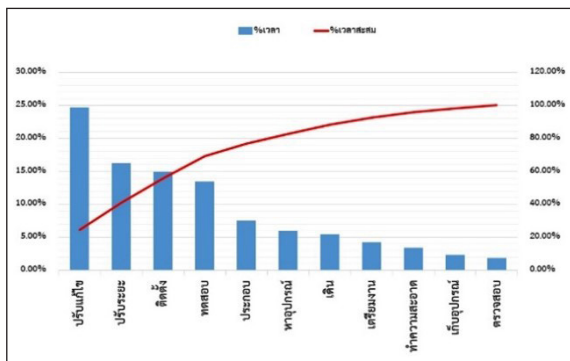
รูปที่ 5 แผนผังพาเรโตแสดงเวลาที่ใช้ในกระบวนการปรับตั้งเครื่องขึ้นรูปกล่อง
