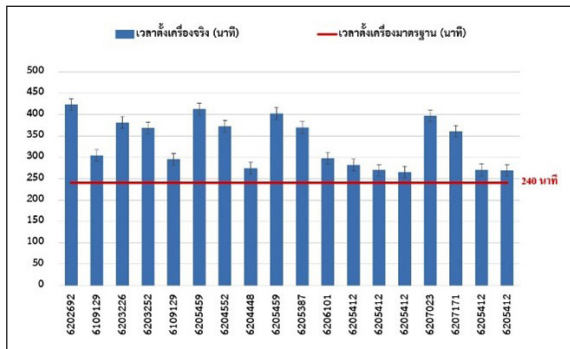
รูปที่ 4 เวลาการปรับตั้งเครื่องกลองลาดฟ้าได้แบบสี่มุม ในช่วงเดือนมกราคม-กรกฎาคม พ.ศ. 2562
