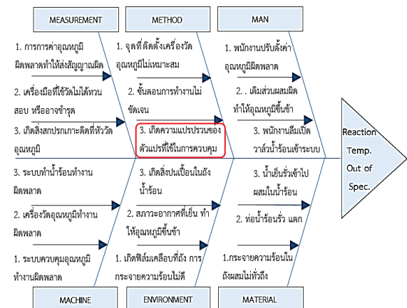
รูปที่ 6 ผังก้างปลาแสดงสาเหตุที่ทำให้อุณหภูมิที่ใช้ทำปฏิกิริยาออกนอกค่าควบคุม
