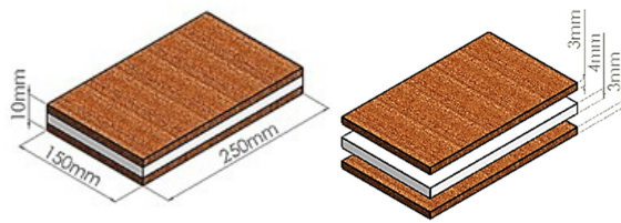
รูปที่ 1 วัสดุแกนผิว 3 ชั้น โดยมีแผ่นประกบด้านบนและล่างจากวัสดุเชิงประกอบพลาสติกและไม้ แกนกลางจากพลาสติก
