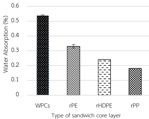
รูปที่ 9 การดูดซับน้ำของชั้นทดสอบวัสดุแซนด์วิช
