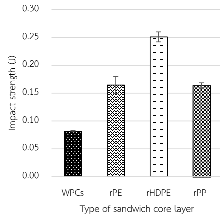
รูปที่ 7 สมบัติการกระแทกของชิ้นทดสอบวัสดุแซนดวิช
