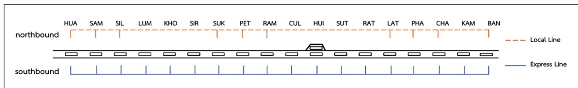
รูปที่ 7 การเดินรถแบบ Express – Normal Operation ในช่วงเวลาเร่งด่วนเย็น 18.00–19.00 น. ทิศทางมุ่งเหนือออกนอกเมือง จากสถานีหัวลำโพงไปยังสถานีบางซื่อ สถานีที่ต้องเพิ่มรางหลักได้แก่สถานีหัวขวง
