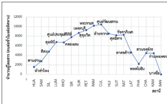
รูปที่ 5 ปริมาณผู้โดยสารสูงสุดในแต่ละตอนเดินรถในช่วงเย็น 18.00-19.00 น. ทิศทางมุ่งเหนือ (Northbound) ออกนอกเมือง จากสถานีหัวลำโพงไปยังสถานีบางซื่อ
