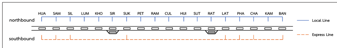
รูปที่ 6 การเดินรถแบบ Express – Normal Operation ในช่วงเวลาเร่งด่วนเช้า 7.00–8.00 น. ทิศทางมุ่งได้เข้าเมือง จากสถานีบางซื่อไปยังสถานีหัวลำโพง สถานีที่ต้องเพิ่มรางหลักได้แก่สถานีศูนย์ประชุมสิริกิติ์ และสถานีรัชดาภิเษก
