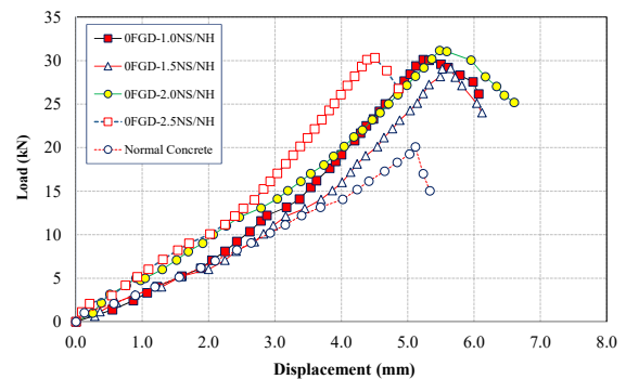
รูปที่ 6 ความสัมพันธ์ระหว่างแรงกระทำกับการเคลื่อนตัวของเหล็กเส้นข้ออ้อยในคอนกรีตโดยใช้เถ้าลอยจีโอพอลิเมอร์มอร์ตาร์ผสมเอฟเจดีบีซีเอ็มร้อยละ 0 เป็นวัสดุเชื่อมประสาน และแปรผันอัตราส่วนสารละลายโซเดียมซิลิเกตต่อโซเดียมไฮดรอกไซด์
