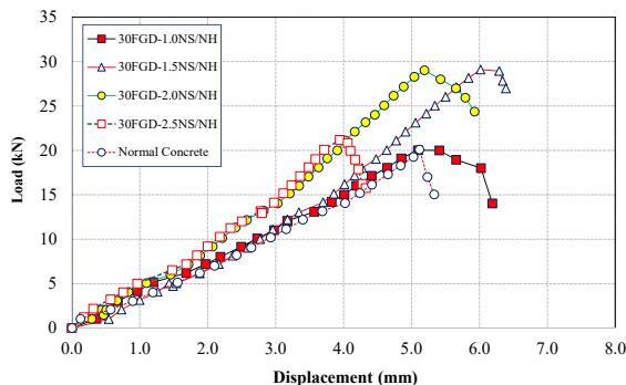
รูปที่ 9 ความสัมพันธ์ระหว่างแรงกระทำกับการเคลื่อนตัวของเหล็กเส้นข้ออ้อยในคอนกรีตโดยใช้เถ้าลอยจีโอพอลิเมอร์มอร์ตาร์ผสมเพฟจีดีบีซีเอ็มร้อยละ 30 เป็นวัสดุเชื่อมประสาน และแปรผันอัตราส่วนสารละลายโซเดียมซิลิเกตต่อโซเดียมไฮดรอกไซด์
