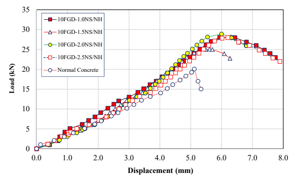
รูปที่ 7 ความสัมพันธ์ระหว่างแรงกระทำกับการเคลื่อนตัวของเหล็กเส้นข้ออ้อยในคอนกรีตโดยใช้เถ้าลอยจีโอพอลิเมอร์มอร์ตาร์ผสมเอฟเจดีบีซีเอ็มร้อยละ 10 เป็นวัสดุเชื่อมประสาน และแปรผันอัตราส่วนสารละลายโซเดียมซิลิเกตต่อโซเดียมไฮดรอกไซด์
