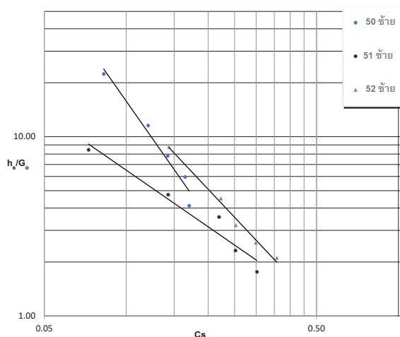
(ก) ความสัมพันธ์ระหว่าง C_s และ h_s/G_0 ของคลองสายย่อย 50L, 51L และ 52L
