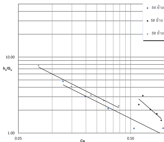
(ข) ความสัมพันธ์ระหว่าง C_s และ h_s/G_0 ของคลองสายย่อย 54L, 58L และ 59L
