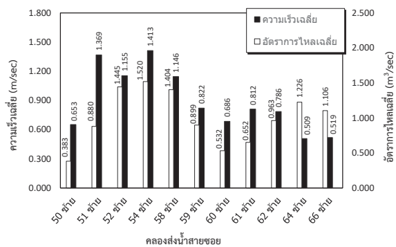
รูปที่ 5 ความเร็วและปริมาณน้ำที่ผ่านหน้าตัดในคลอง
