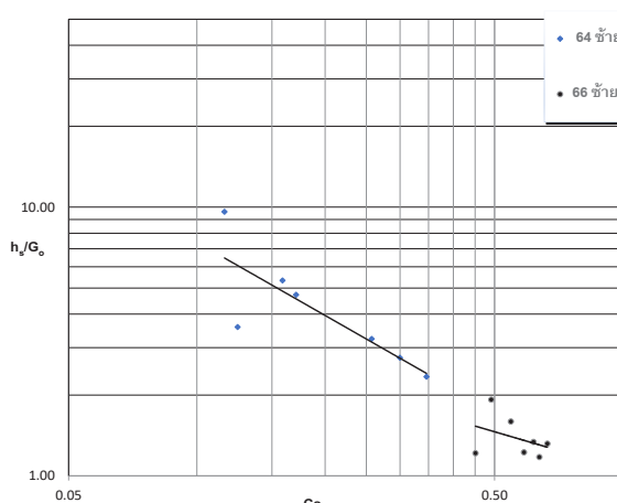
(ง) ความสัมพันธ์ระหว่าง C_s และ h_s/G_0 ของคลองสายย่อย 64L และ 66L
