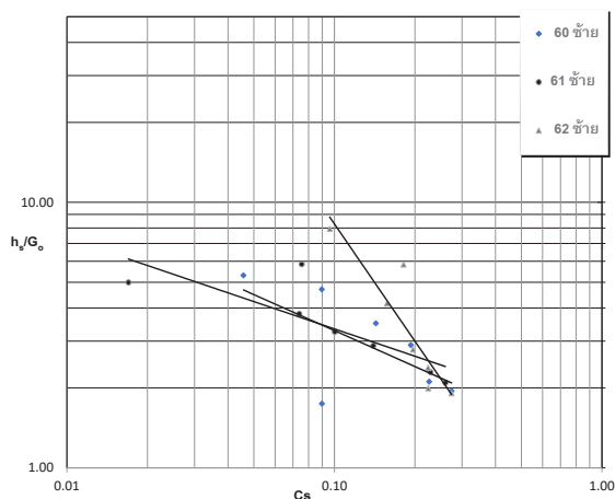
(ค) ความสัมพันธ์ระหว่าง C_s และ h_s/G_0 ของคลองสายย่อย 60L, 61L และ 62L
