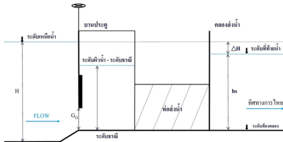
รูปที่ 4 ลักษณะการไหลของน้ำลอดใต้บ้านตรงแบบท่วม ท้ายบานระบายน้ำ
