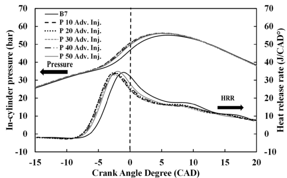
รูปที่ 3 ค่าความดันในกระบอกสูบและอัตราการปลดปล่อยความร้อน ปรับตั้งองศาการฉีดที่ -16.5 CAD
