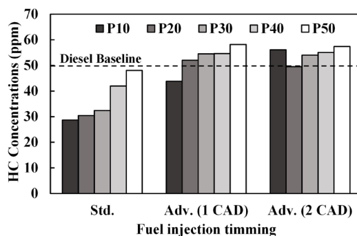
รูปที่ 8 ปริมาณไฮโดรคาร์บอนในไอเสียที่การปรับตั้งองศาฉีดที่ -16.5 CAD และ -17.5 CAD
