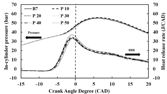
รูปที่ 2 ค่าความดันในกระบอกสูบและอัตราการปลดปล่อยความร้อน
