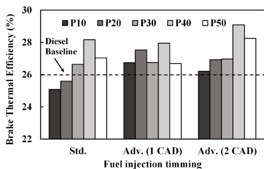
รูปที่ 7 ประสิทธิภาพเชิงความร้อนเบรกที่การปรับตั้งองศาฉีดที่ -16.5 CAD และ -17.5 CAD
