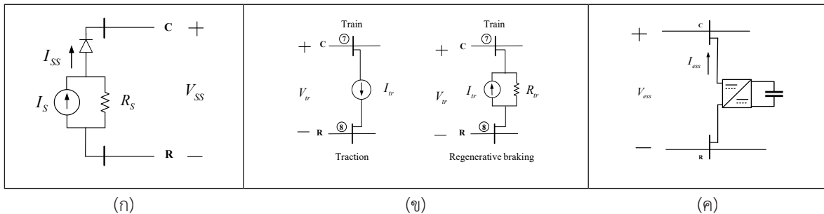
รูปที่ 4 แบบจำลองในระบบไฟฟ้า (ก) แบบจำลองสถานีไฟฟ้าขับเคลื่อน (ข) แบบจำลองรถไฟฟ้า (ค) แบบแบบจำลองระบบเก็บสะสมพลังงานแบบบริมทาง
