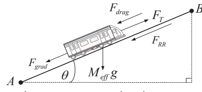
รูปที่ 2 แผนภาพการเคลื่อนที่ของรถไฟฟ้า
