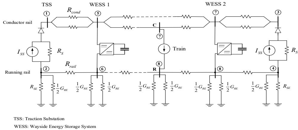
รูปที่ 3 ระบบไฟฟ้าขับเคลื่อนแบบ Multi-conductor System
