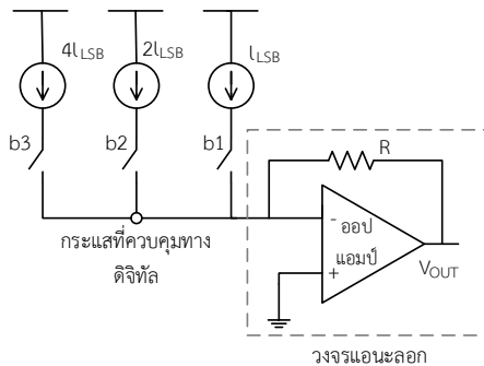
รูปที่ 1 ตัวอย่างการใช้วงจร DAC แบบกระแสขนาด 3 บิต เพื่อสร้างกระแสที่ควบคุมทางดิจิทัลป้อนเข้าวงจรแอนะล็อก
