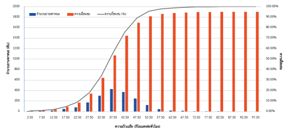
รูปที่ 12 ความถี่สะสมและความเร็วของยานพาหนะที่ 85 เพอร์เซ็นต์ไทล์ บนถนนตากสินมหาราชในช่วงเวลาไม่เร่งด่วน (45 กิโลเมตรต่อชั่วโมง)
