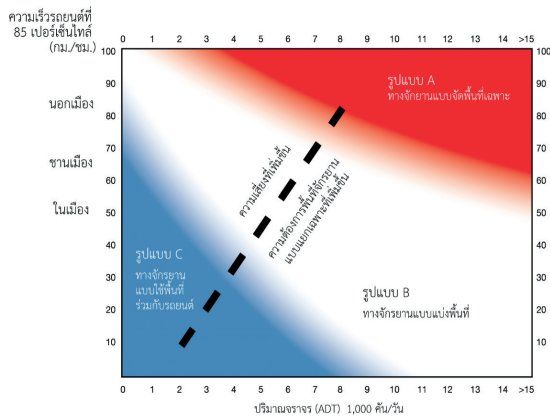
รูปที่ 5 แผนภูมิระหว่างความเร็วรถที่ 85 เปอร์เซ็นต์ไทล์ (Y) และปริมาณจราจร (AADT) 1,000 คันต่อวัน (X) [7]
