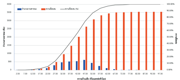
รูปที่ 13 ความถี่สะสมและความเร็วของยานพาหนะที่ 85 เพอร์เซ็นต์ไทล์ บนถนนจันทอุดมในช่วงเวลาเร่งด่วน (50 กิโลเมตรต่อชั่วโมง)
