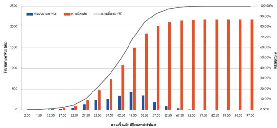
รูปที่ 14 ความถี่สะสมและความเร็วของยานพาหนะที่ 85 เปอร์เซ็นไทล์ บนถนนจันทอุดมในช่วงเวลาไม่เร่งด่วน (55 กิโลเมตรต่อชั่วโมง)
