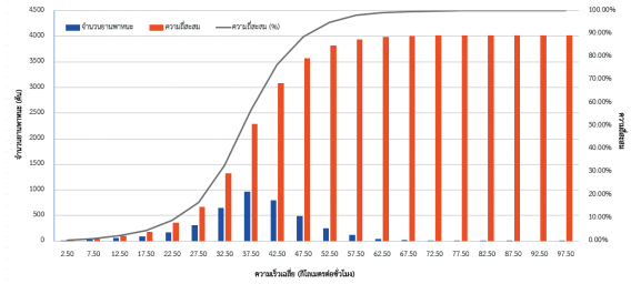
รูปที่ 11 ความถี่สะสมและความเร็วของยานพาหนะที่ 85 เพอร์เซ็นต์ไทล์ บนถนนตากสินมหาราชในช่วงเวลาเร่งด่วน (40 กิโลเมตรต่อชั่วโมง)
