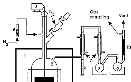
รูปที่ 5 กระบวนการไมโครเวฟไพโรไลซิสโดยใช้พลาสติกที่ใช้แล้วเป็นสารตั้งต้น [11] โดย 1. เตาไมโครเวฟ 2. ถังปฏิกรณ์ 3. มอเตอร์ 4. วาล์วควบคุมก๊าซเฉื่อย ( \text{N}_2 ) 5. โรตารีมอเตอร์ 6. ขวดปริมาตร (Flask) 7. คอนเดนเซอร์ 8,9. ตัวดักจับก๊าซ 10. ตัวกรองละเอียด [11]
