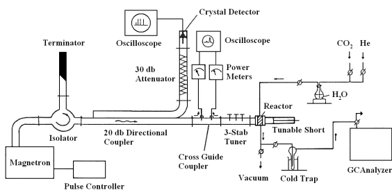
รูปที่ 6 กระบวนการไมโครเวฟไพโรไลซิสโดยใช้เบนซีน (Benzene) เป็นสารตั้งต้น [18]
