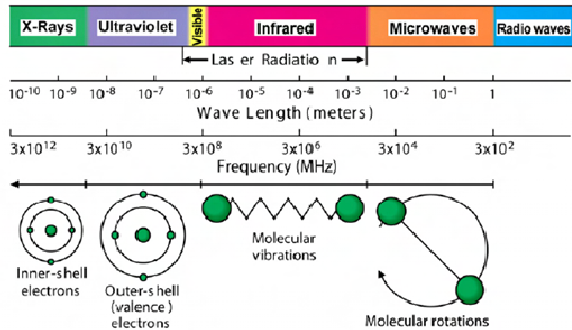
รูปที่ 1 ภาพแสดงสเปกตรัมคลื่นแม่เหล็กไฟฟ้าในช่วงความถี่ต่างๆ [1]
