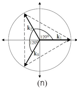
รูปที่ 3 เวกเตอร์ k_1, k_2 และ k_3 ที่ทำมุมต่อกันเท่ากับ 120^\circ
