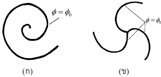
รูปที่ 14 (ก) เส้นเวียนกันหอยแบบ 1 แขน (ข) เส้นเวียนกันหอยแบบ 3 แขน [12]
