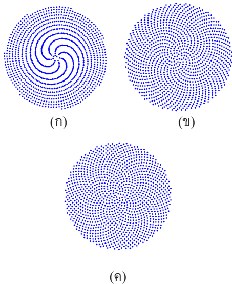
รูปที่ 12 เมล็ดดอกทานตะวันที่เกิดขึ้นใหม่ เมื่อถูกบรรจุด้วยมุม (ก) \phi = 360^\circ \pi (ข) \phi = 360^\circ \sqrt{2} และ (ค) \phi \approx 137.5^\circ ตามลำดับ
