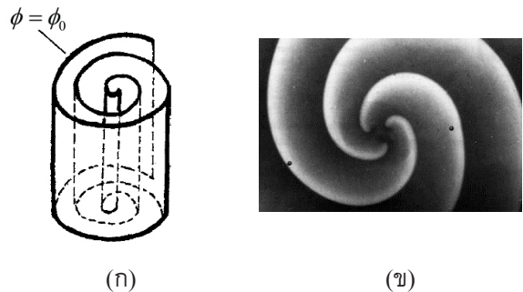
รูปที่ 13 (ก) เส้นเวียนกันหอยใน 3 มิติ (ข) เส้นเวียนกันหอยใน 3 มิติที่เกิดขึ้นจากการทดลองของปฏิกิริยา
