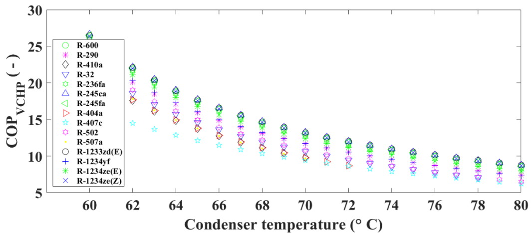
รูปที่ 9 สัมประสิทธิ์สมรรถนะการทำความร้อนของระบบปั๊มความร้อน เมื่ออุณหภูมิด้านเครื่องควบแน่นมีอุณหภูมิต่าง ๆ
