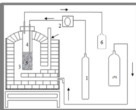
(ข) เครื่องดันแบบเตาเผาอุณหภูมิสูง
