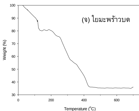
รูปที่ 5 การสลายตัวทางความร้อนของชีวมวล
