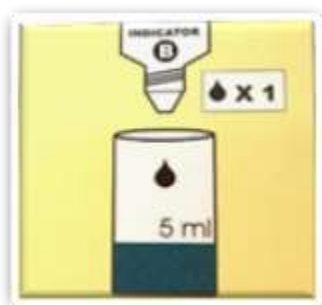
รูปที่ 12 ขั้นที่ 2 หยดอินดิเคเตอร์ B จำนวน 1 หยด แล้วเขย่าให้เข้ากัน น้ำตัวอย่างจะเปลี่ยนเป็นสีฟ้าอมเขียว [5]
