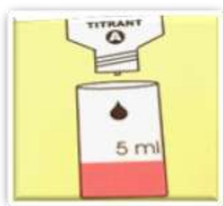
รูปที่ 14 ขั้นที่ 4 หยดไทเตรนต์ A ลงอีก 1 หยด น้ำตัวอย่างจะเปลี่ยนเป็นสีชมพูจำนวน หยดทั้งหมดแล้วคูณ 17 จะได้ผลเป็นค่าสภาพความเป็นด่างรวม [5]
