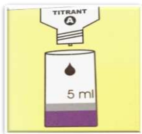
รูปที่ 13 ขั้นที่ 3 หยดไทเตรนต์ A ลงในน้ำตัวอย่างทีละหยดช้า ๆ พร้อมทั้งเขย่าให้เท่ากัน จนสีของน้ำตัวอย่างเปลี่ยนเป็นสีเทาอมม่วง [5]
