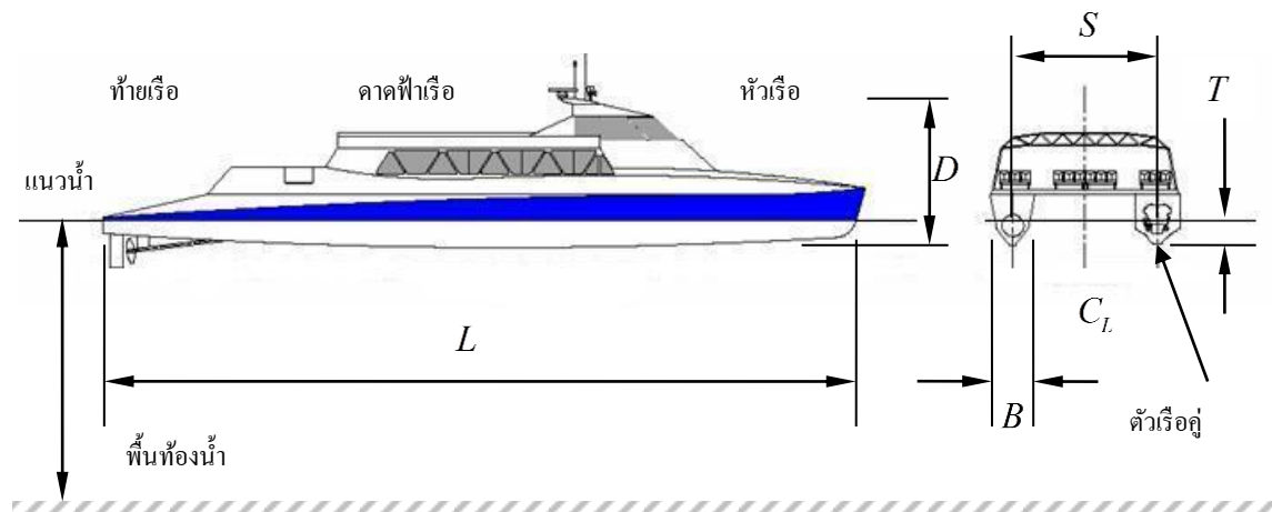
รูปที่ 1 เรือแบบตัวเรือคู่ (Catamaran)
