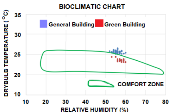
รูปที่ 3 กราฟแสดงสภาวะน่าสบาย
