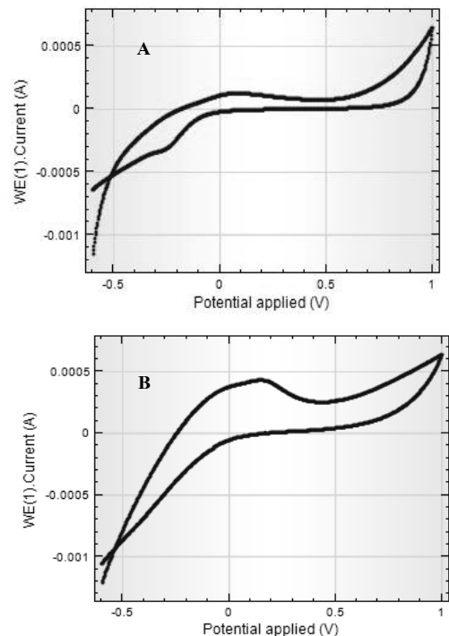
รูปที่ 5 (A) ไชคลิกโวลแทมเมทรีของของเสียกลีเซอรอล และ (B) ไชคลิกโวลแทมเมทรีของน้ำเสียโรงงานฟอกหนัง
