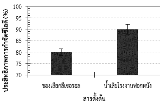
รูปที่ 2 แสดงประสิทธิภาพการกำจัดชีโอดีจากของเสียกลีเซอรอลและน้ำเสียโรงงานฟอกหนัง
