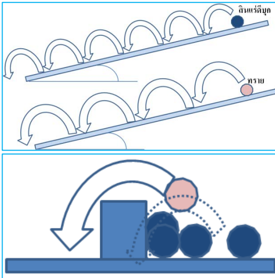
รูปที่ 3 บน) การเคลื่อนไหวยของเม็ดแร่ดิบและเม็ดแร่ทรายบนพื้น โตะสั่นที่มีความเอียง (ล่าง) สิ้นแร่ดิบที่ถูกดูดขึ้นซึ่งสะสมตัวและการเคลื่อนตัวของเม็ดทรายที่เหยียบสิ้นแร่ดิบข้ามแนวลูกขึ้นได้
