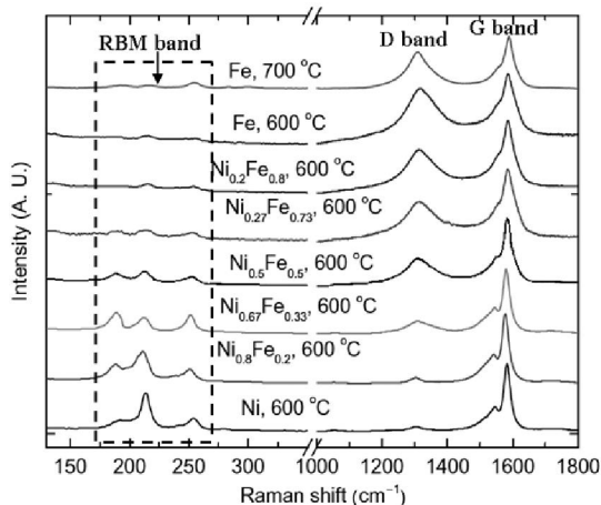
รูปที่ 7 เปรียบเทียบท่อนาโนคาร์บอนที่สังเคราะห์ได้จากการวิเคราะห์ด้วยเครื่อง Raman โดยการแปรค่าสัดส่วนของตัวเร่งปฏิกิริยา Ni กับ Fe ( \text{Ni}_x\text{Fe}_{1-x} ) ที่ 600^{\circ}\text{C} และ Fe ที่ 700^{\circ}\text{C} [19]
