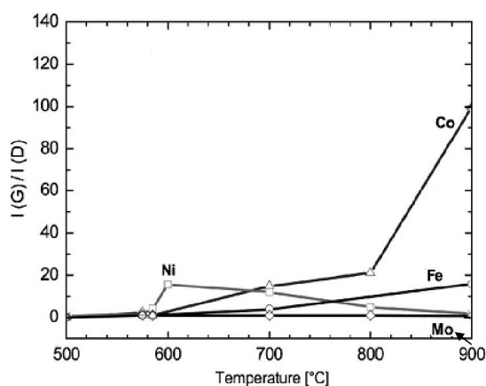
รูปที่ 6 เปรียบเทียบสัดส่วนของ G และ D bands ( I_G/I_D ) ในการสังเคราะห์ท่อนาโนคาร์บอนโดยใช้ตัวเร่งปฏิกิริยา Co, Ni, Fe และ Mo ที่อุณหภูมิ 500^{\circ}\text{C} ถึง 900^{\circ}\text{C} [16]
