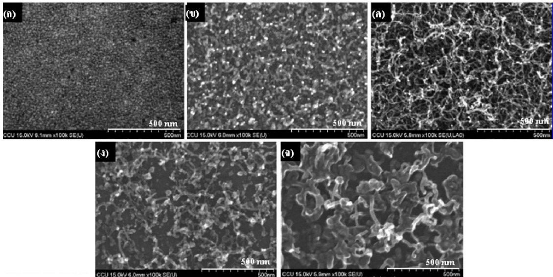
รูปที่ 5 ภาพถ่าย FESEM แสดงการเกิด CNTs บนพื้นผิวตัวรองรับ Si ที่มี \text{Ni}(\text{NO}_3)_2 เป็นตัวเร่งปฏิกิริยา โดยใช้เปลวไฟของ บิวเทน (butane) ที่อุณหภูมิ 880^\circ\text{C} และแปรค่าเวลาในการสังเคราะห์ (ก) 3 วินาที (ข) 5 วินาที (ค) 10 วินาที (ง) 20 วินาที (จ) 40 วินาที [14]
