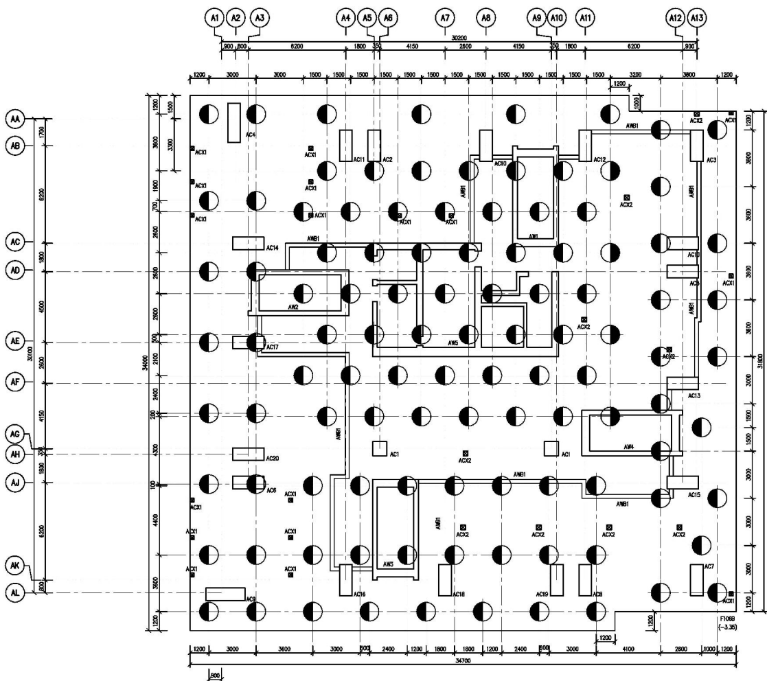
รูปที่ 1 แผนฐานรากคอนกรีต
