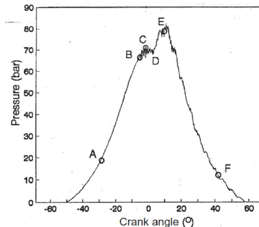
รูปที่ 1 ความสัมพันธ์ระหว่างความดันในห้องเผาไหม้กับเพลวข้อเหวี่ยงในเครื่องยนต์พลังงานร่วม [7]
