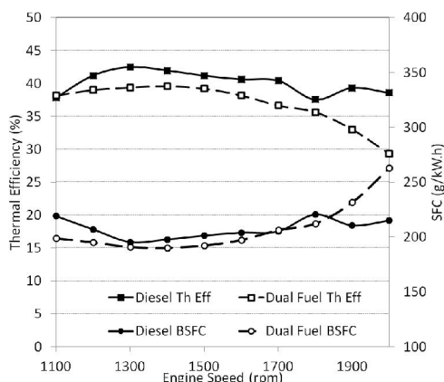
รูปที่ 8 การเปรียบเทียบประสิทธิภาพเชิงความร้อนและอัตราการสิ้นเปลืองเชื้อเพลิงเฉพาะของเครื่องยนต์
