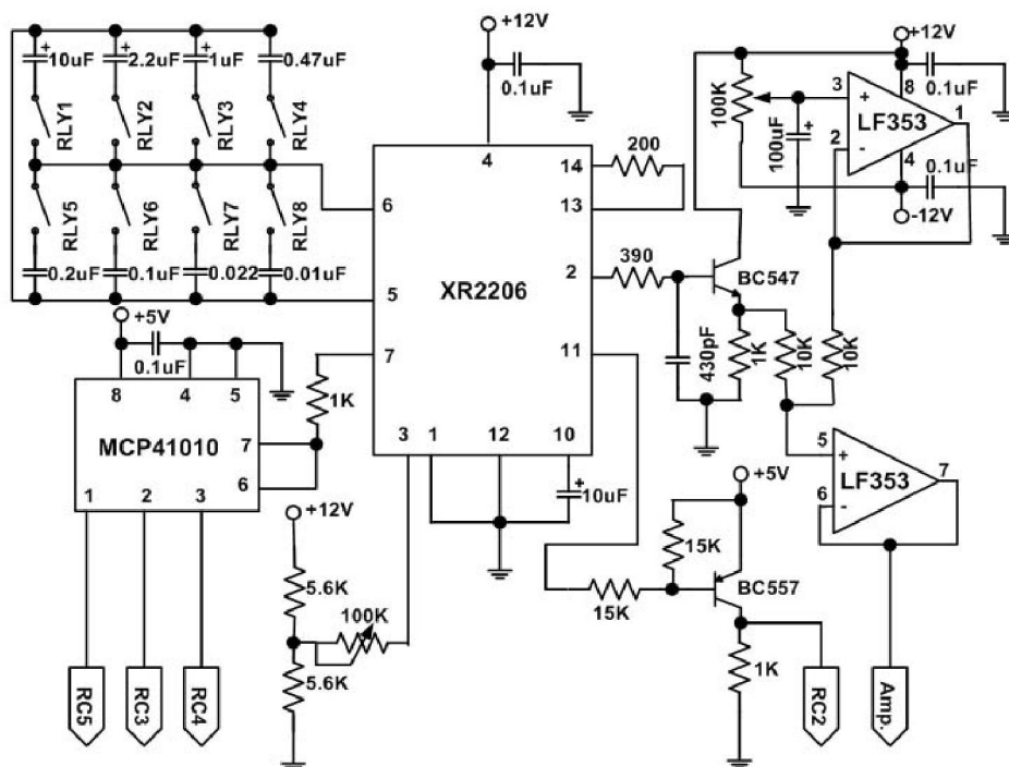
รูปที่ 3 วงจรกำเนิดสัญญาณ
