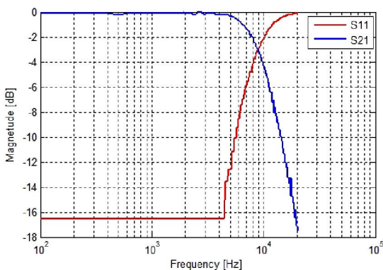
รูปที่ 11 ผลตอบสนองทางความถี่วงจรกรองความถี่ต่ำ
