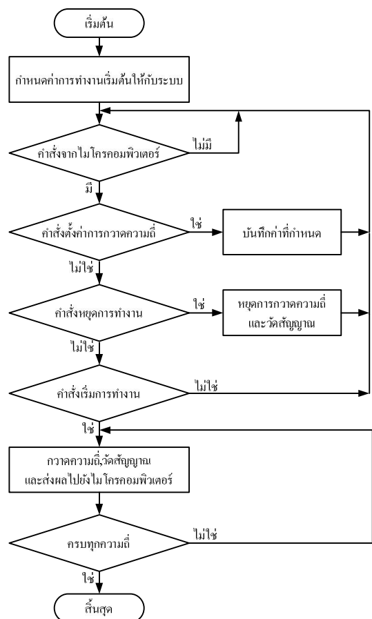
รูปที่ 7 ฟังก์ชัน โปรแกรมชุดการวัดใช้ไมโครคอนโทรลเลอร์
