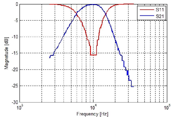
รูปที่ 12 ผลตอบสนองทางความถี่วงจรกรองความถี่แถบผ่าน
