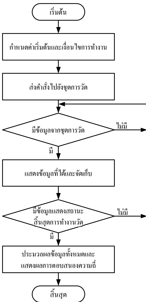
รูปที่ 6 ฟังก์ชัน โปรแกรมการวิเคราะห์โครงข่ายเสมือนจริง
