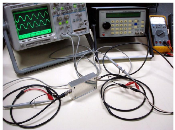
รูปที่ 13 การวัดวงจรกรองความถี่ด้วยเครื่องมือวัด
