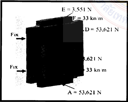
รูปที่ 5 ตำแหน่งของแรงกระทำที่ Saddle
