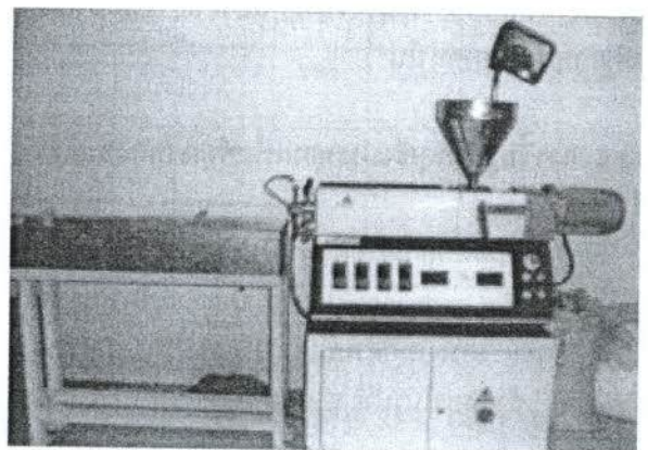
รูปที่ 4 เครื่องอัดรีดแบบเกลียวนอนเดี่ยว (Lab Tech Engineering)
