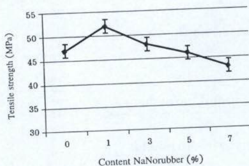
รูปที่ 5 ค่าการต้านทานแรงดึง (Tensile strength)
