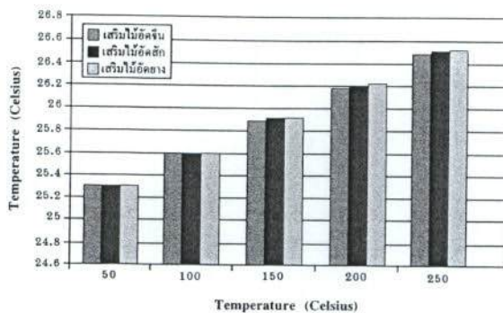
รูปที่ 8 การเปรียบเทียบผลการจำลองไฟในเคโอลิเมนต์ของวัสดุแกนวิชรังผึ้งเสริมไม้อัดทั้งสามชนิด
