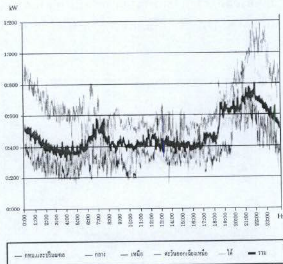
รูปที่ 4 Load Profile ของบ้านอยู่อาศัยกลุ่มที่มีปริมาณการใช้พลังงานไฟฟ้ามากกว่า 150 หน่วยต่อเดือนทั่วประเทศ แยกตามรายการ (วันทำงาน จันทร์ - ศุกร์)
