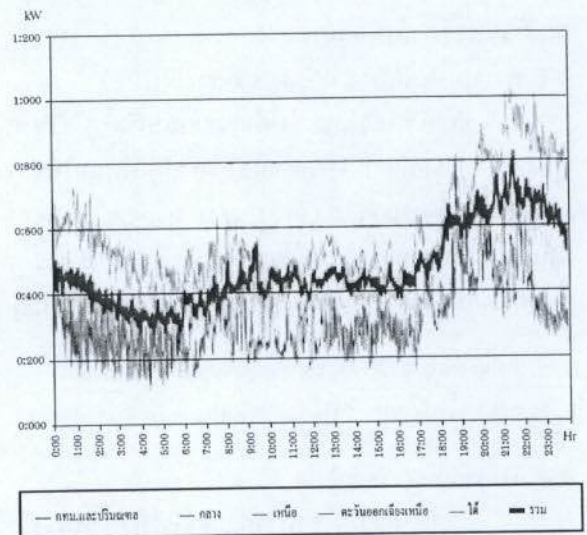
รูปที่ 5 Load Profile ของบ้านอยู่อาศัยกลุ่มที่มีปริมาณการใช้พลังงานไฟฟ้ามากกว่า 150 หน่วยต่อเดือนทั่วประเทศ แยกตามรายการ (วันหยุด เสาร์-อาทิตย์)
