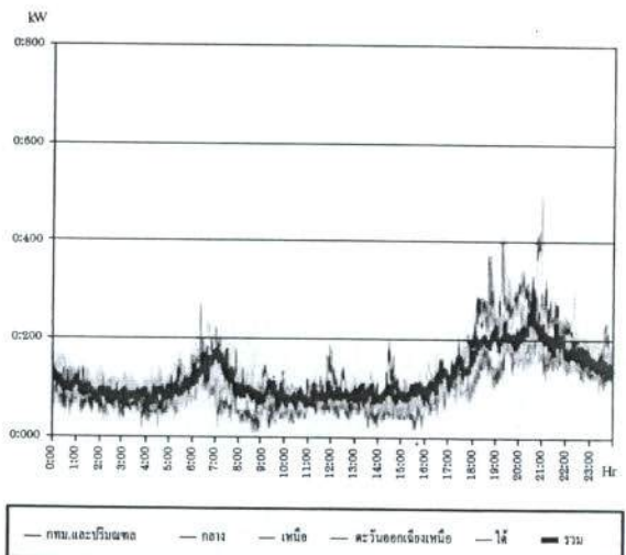
รูปที่ 2 Load Profile ของบ้านอยู่อาศัยกลุ่มที่มีปริมาณการใช้พลังงานไฟฟ้าไม่เกิน 150 หน่วยต่อเดือนทั่วประเทศ แยกตามรายภาค (วันทำงาน จันทร์ - ศุกร์)
