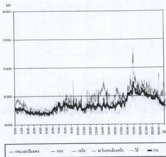
รูปที่ 3 Load Profile ของบ้านอยู่อาศัยกลุ่มที่มีปริมาณการใช้พลังงานไฟฟ้าไม่เกิน 150 หน่วยต่อเดือนทั่วประเทศ แยกตามรายการ (วันหยุด เสาร์-อาทิตย์)
