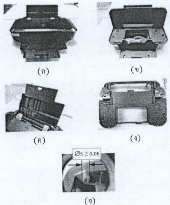
รูปที่ 1 รายละเอียดของชิ้นงานและจุดปัญหา
