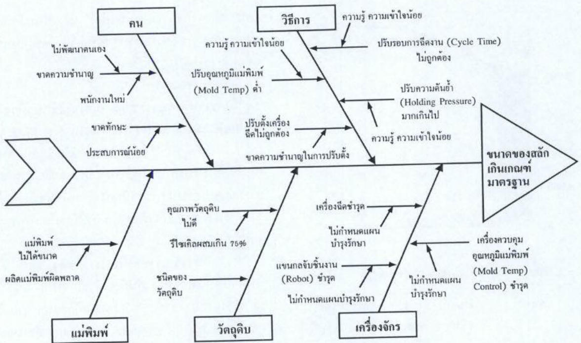
รูปที่ 3 การวิเคราะห์สาเหตุของสลัก เกินเกณฑ์มาตรฐานโดยแผนภูมิแก๊งปลา
